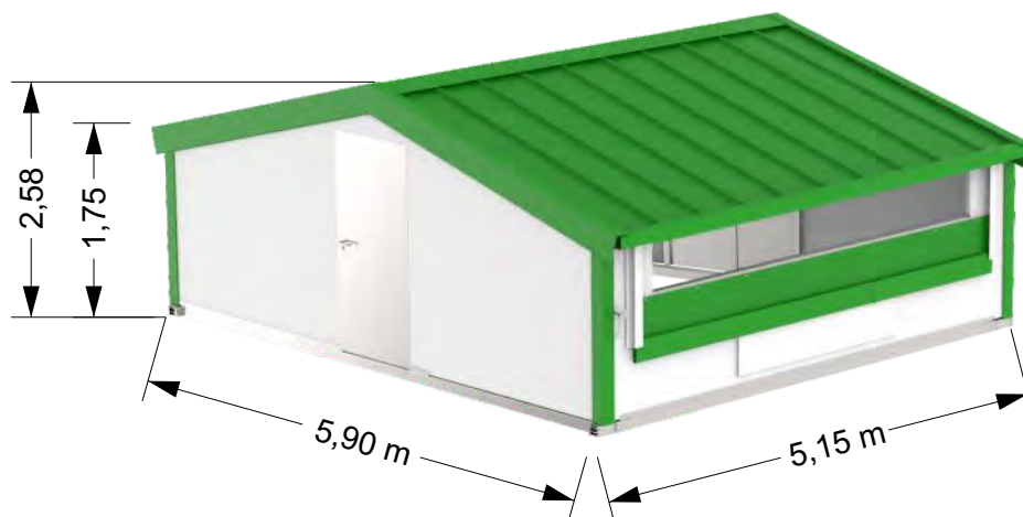
Cod. 30112 Bâtiment en toile. Cod. 30113 Bâtiment avec treillis.
