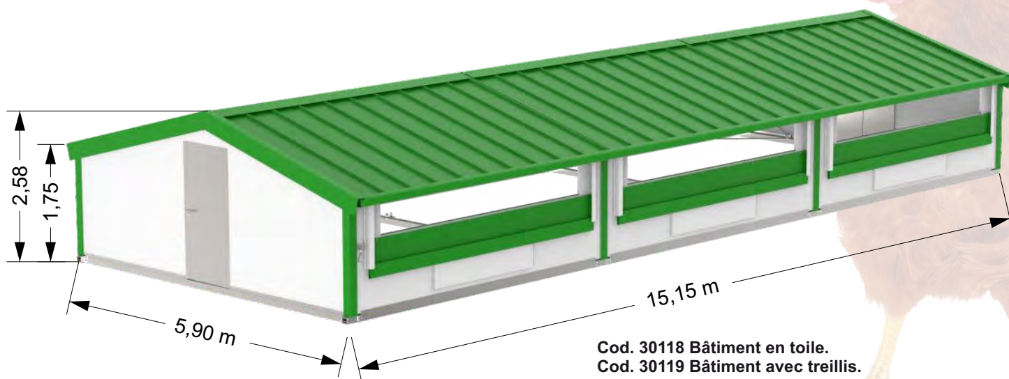
Cod. 30116 Bâtiment en toile. Cod. 30117 Bâtiment avec treillis.
